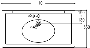
Royal Consolle Calipso Calipso Consolle Consola Calipso COD. 30060
