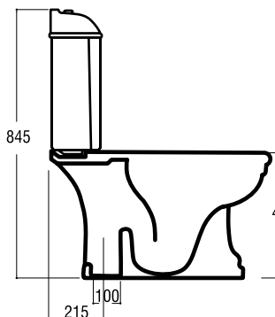
Royal Coprivaso Seat cover Asiento □ COD. 27050 ■ COD. 27052 (legno/wood/madera)
