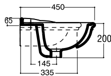
Royal Consolle Calipso Calipso Consolle Consola Calipso COD. 30060
