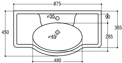
Royal Consolle cm 85 Consolle cm 85 Consola cm 85 COD. 30355
