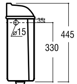
Royal Set per cassetta alta (cat+mecc+ tubo) Set for high cistern (pipe+chain+mechanism) Set para tanque alto (tubo+cad+mecc) ■ COD. 40166 acciaio/chrome/cromo ■ COD. 40167 bronzo/bronze/bronze
