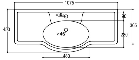
Royal Consolle cm 105 Consolle cm 105 Consola cm 105 COD. 40127
