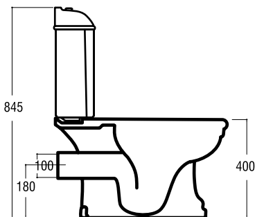
Royal Vaso monoblocco scarico P Wc bowl monobloc wall trap Inodoro para tanque bajo salida H COD. 27001
