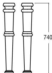
Royal Kit coppia di piedini per consolle cm 110 e calipso/ Kit pair of legs for consolle cm 110 and calipso/ Kit pareja patas para consola cm 110 y calipso COD. 40191
