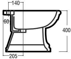
Royal Bidet Bidet COD. 27040
