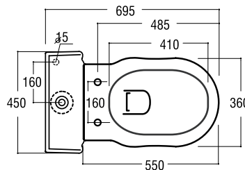
Royal Vaso monoblocco scarico S Wc bowl monobloc floor trap Inodoro para tanque bajo salida V COD. 27002
