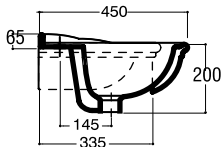
Royal Consolle cm 85 Consolle cm 85 Consola cm 85 COD. 30355
