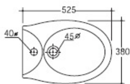
Hola Bidet sospeso Wall hanging bidet Bidé suspendido COD. 29042
