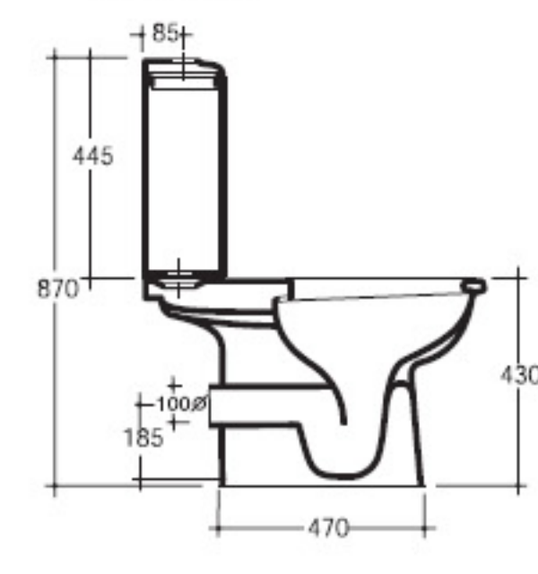
Hola Vaso monoblocco scarico S Wc bowl monobloc floor trap Inodoro para tanque bajo salida V COD. 29002
