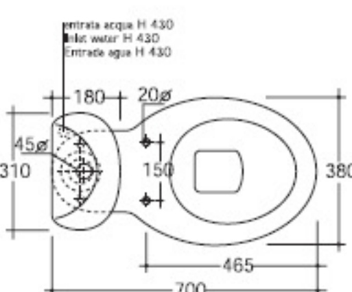
Hola Cassetta monoblocco Wc cistern monobloc Tanque bajo COD. 29014
