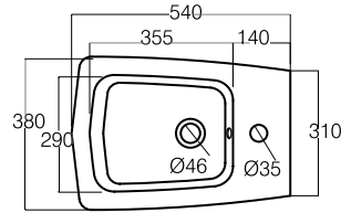
Oceano Bidet Bidet Bidé COD. 30332
