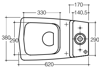
Oceano Vaso monoblocco scarico S/P Wc bowl monobloc F/W trap Inodoro para tanque bajo salida V/H COD. 30424
