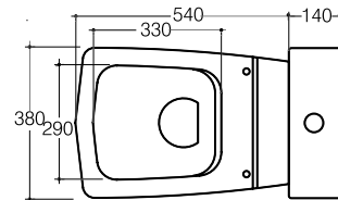
Kit Totem Hard - Meccanismo Geberit Kit Totem Hard - Geberit Mechanism Kit Totem Hard - Mecanismo Geberit □ COD. 40201 ■ COD. 40202
