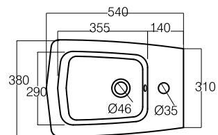
Oceano Bidet sospeso Wall hanging bidet Bidé suspendido COD. 30334
