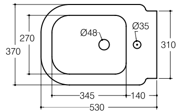
D-Style Bidet Bidet Bidé COD. 40035
