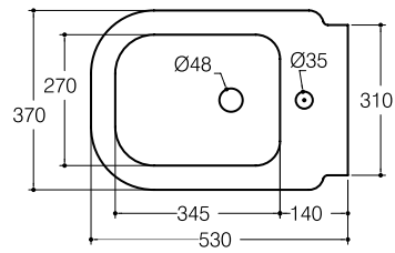
D-Style Bidet sospeso Wall hanging bidet Bidé suspendido COD. 40036
