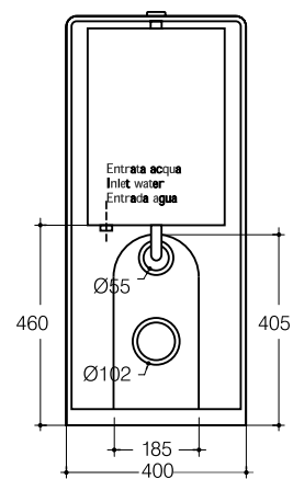
D-Style Vaso scarico S/P Wc bowl F/W trap Inodoro Salida V/H □ COD. 40031
